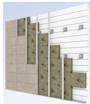
Hinterlüftete Fassade
