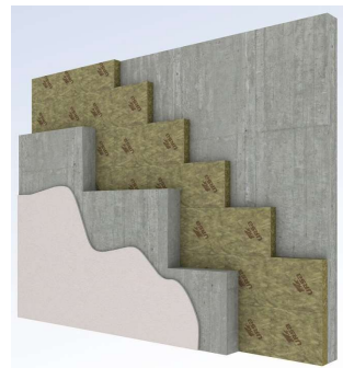
Gebäudetrennwand / Liftschacht
