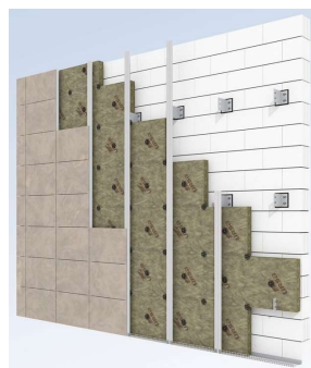
Hinterlüftete Fassade
